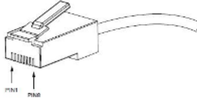
Şekil 3-3 Konsol bağlantı noktasının RJ45 bağlacı
