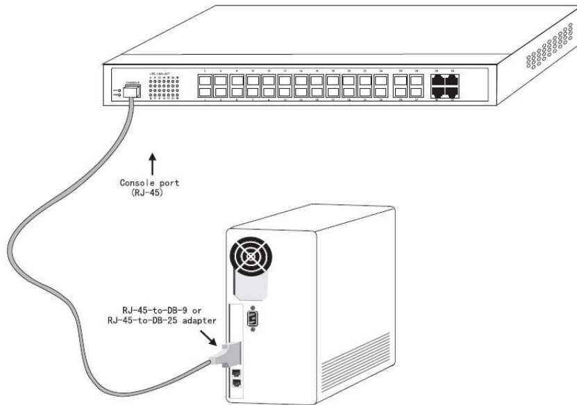
Şekil 3-4 BDCOM S2528GX ve bilgisayarın konsol portunun bağlanması
