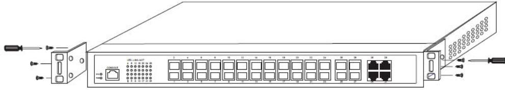
Şekil 3- 1 Anahtarın kutuya sabitleme
