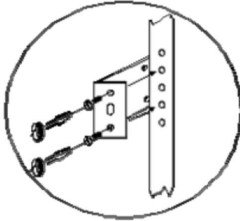
Şekil 3-2 Anahtarın dolabın üzerine monte edilmesi
