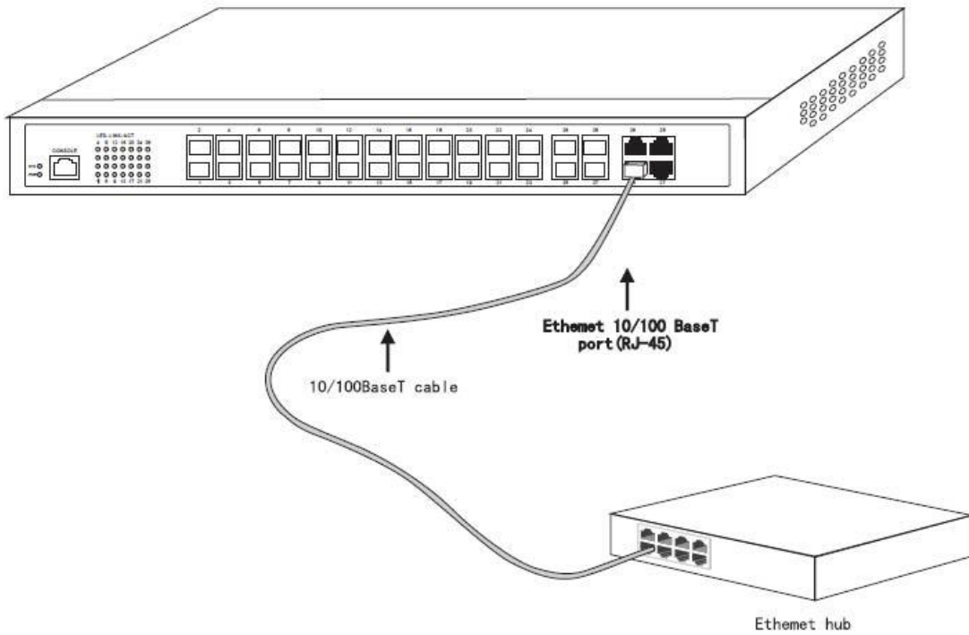
Şekil 3-8 1000Base-TX portunu ve diğer Ethernet terminallerini bağlama
