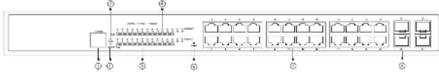
Şekil 1- 1 S2528PB anahtarının ön şablonu
