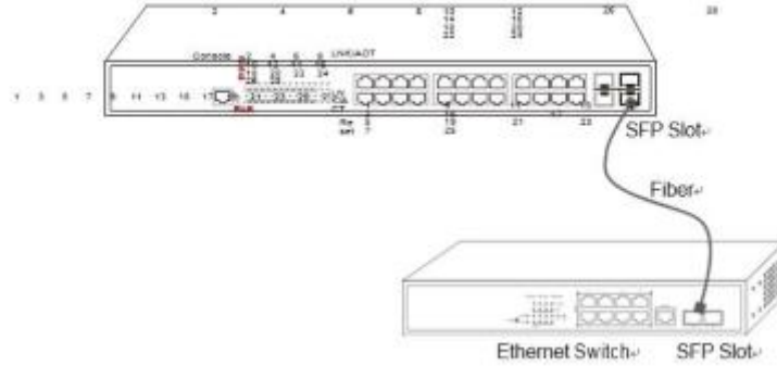
Şekil 3-6 SFP portunu ve diğer Ethernet terminallerini bağlama
