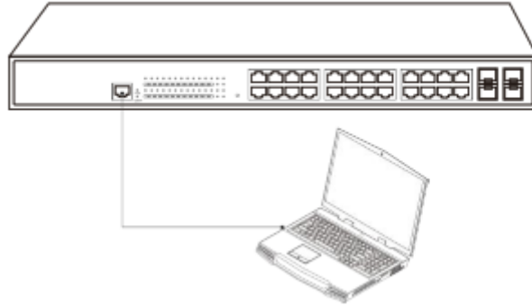
Şekil 3-4 Konsol bağlantı noktasındaki kablo bağlantısı
