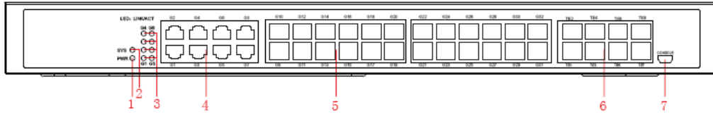
Şekil 1- 1 S3740F anahtarının ön şablonu
