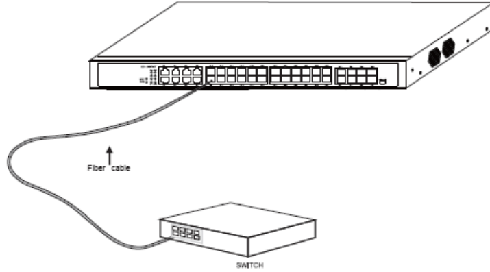
Şekil 3-9 1000 SFP portunu ve diğer Ethernet terminallerini bağlama
