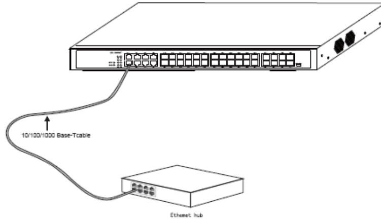
Şekil 3-8 1000Base-TX portunu ve diğer Ethernet terminallerini bağlama
