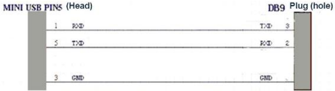
Şekil 3-4 Konsol bağlantı noktasındaki kablo bağlantısı
