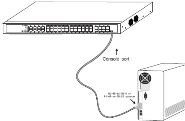
Şekil 3-4 Konsol bağlantı noktasındaki kablo bağlantısı
