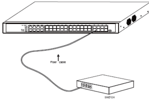
Şekil 3-6 10G SFP + bağlantı noktaları diğer Ethernet terminal cihazlarına bağlanır
