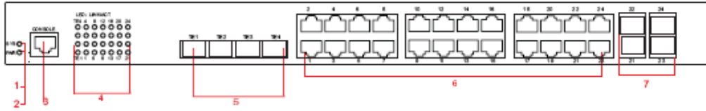
Şekil 1- 1 S2928 anahtarının ön şablonu
