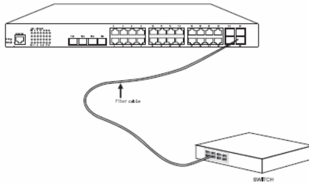
Şekil 3-8 SFP portunu ve diğer Ethernet terminallerini bağlama
