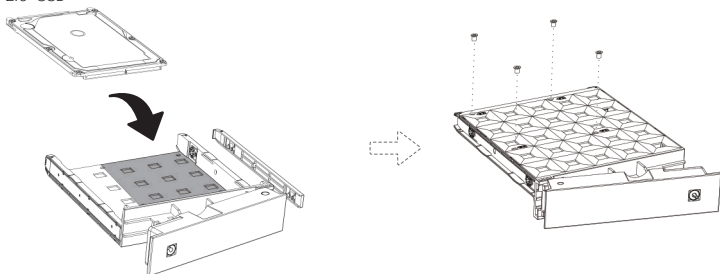
2.5" SSD
